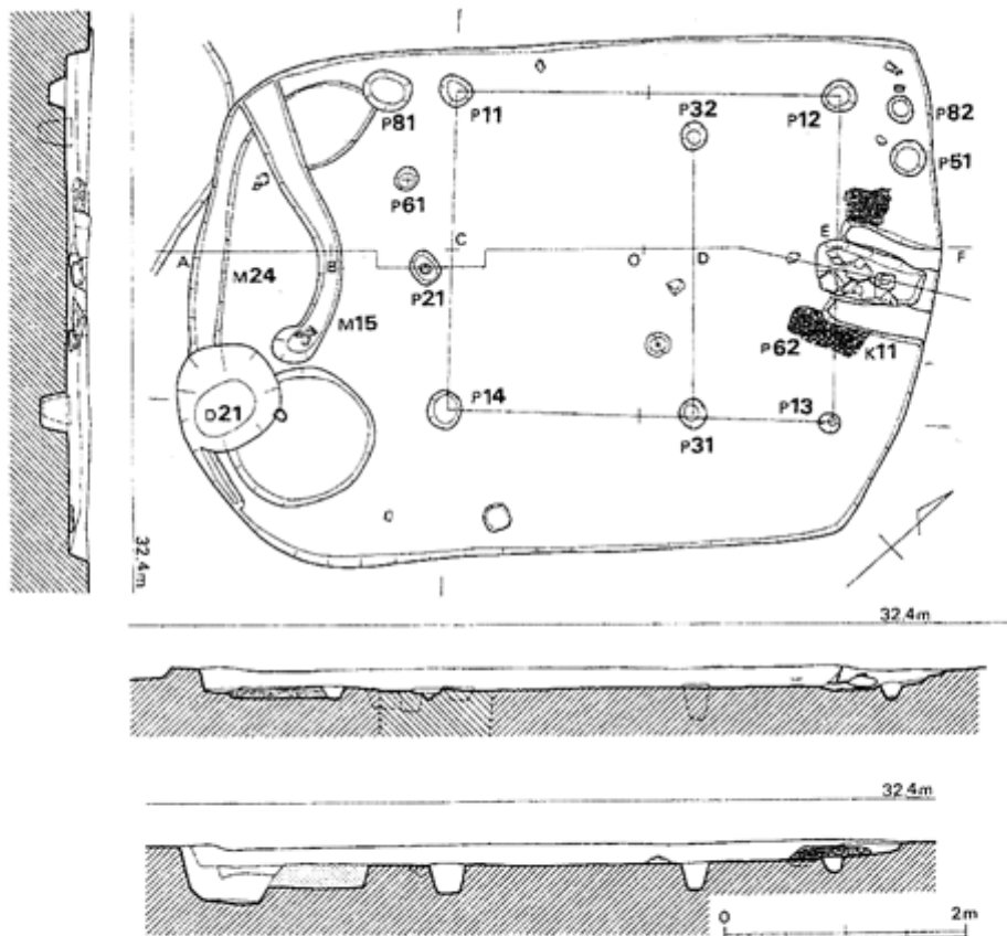
6号住居跡実測図 (1/60)
