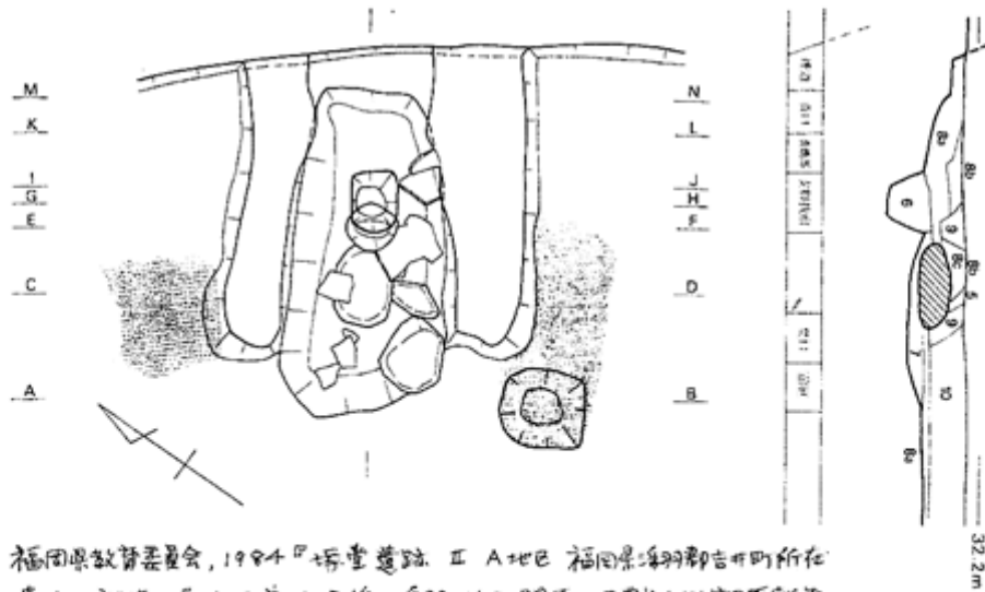
6号住居跡実測図 (1/60)
